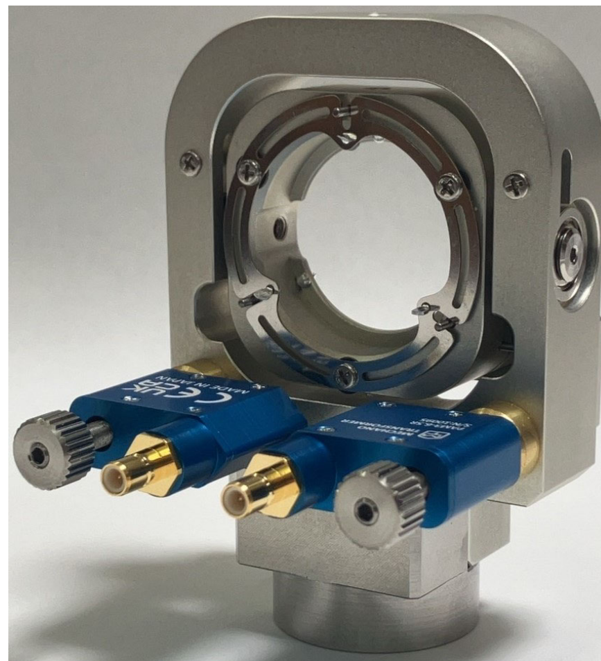
アクチュエータは有限会社メカノトランスフォーマ社の PAM3-6.5R を搭載
